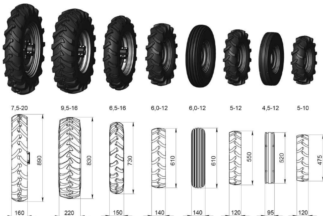
Рис. 18. Размеры колес
