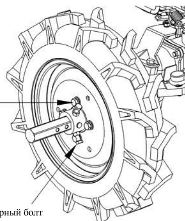
Регулируемая колеса
