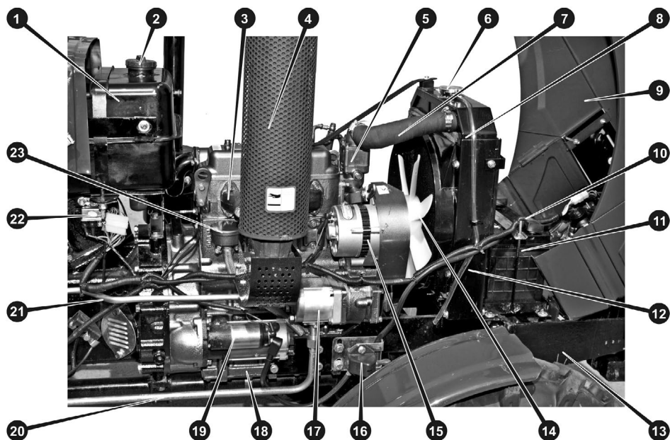
Рисунок 3.5. Двигатель LL380BT и KM385BM, вид справа.
