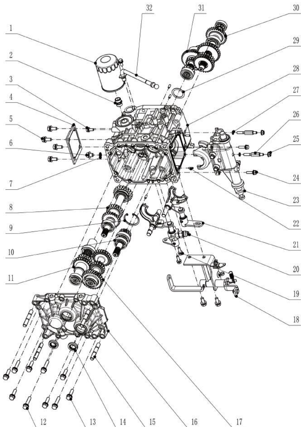
ТА25.37 Коробка передач в сборе 6 передач
