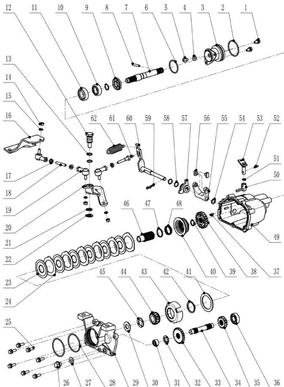
ТА25. 31. 05 Устройство поворота на удвоенной скорости в сборе
