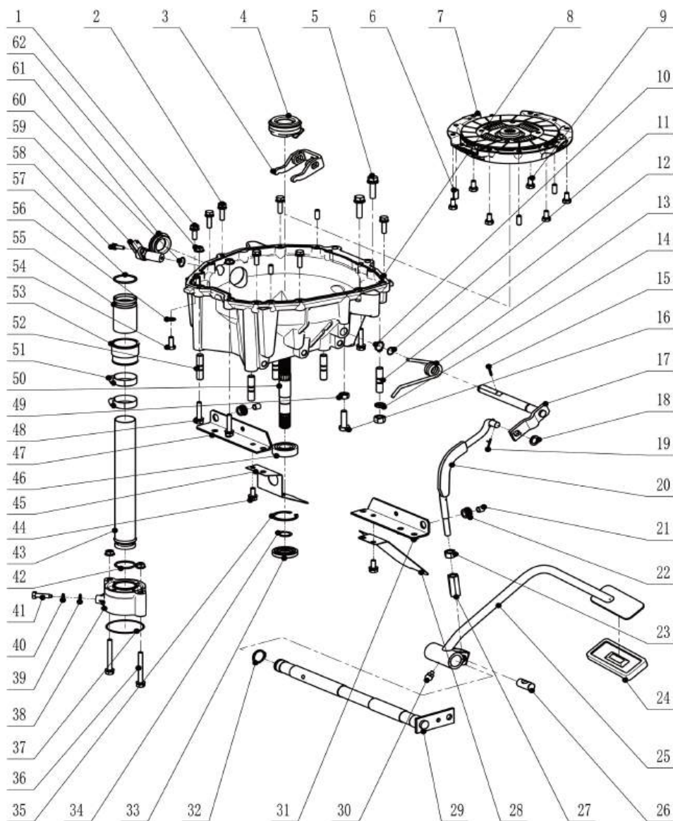
ТА25. 21 Подсборка главного сцепления
