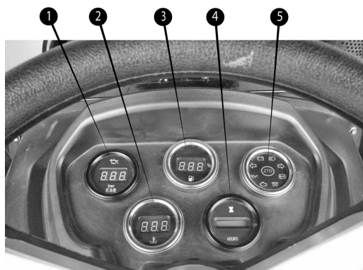
Рисунок 3.8. Панель приборов
