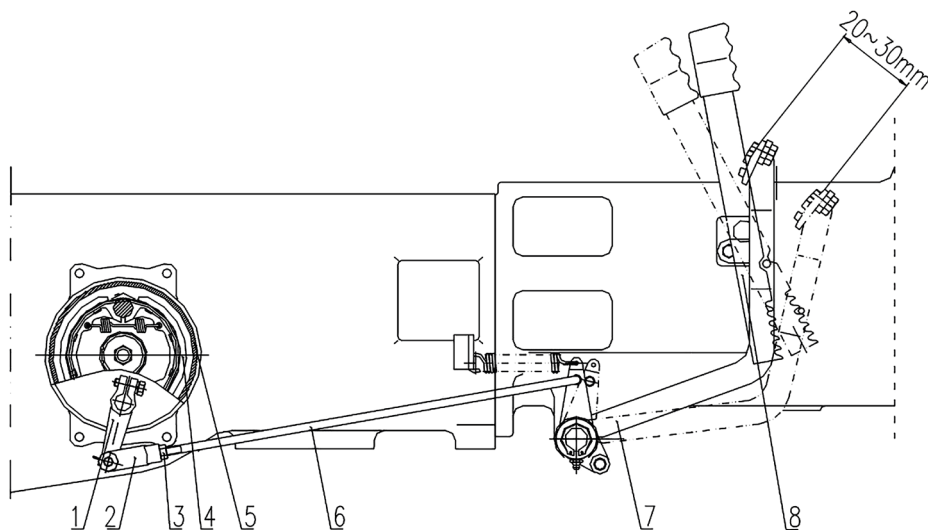
Рис. 5.4 Тормозная система
