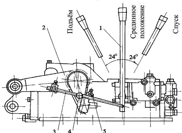
Рис. 5.18 Корректировка опускания
